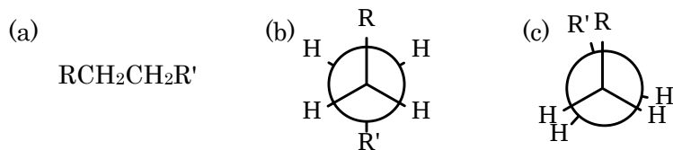
図 \text{RCH}_2\text{CH}_2\text{R}' の立体配座
