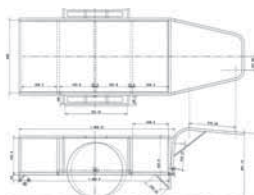
リヤカー図面
